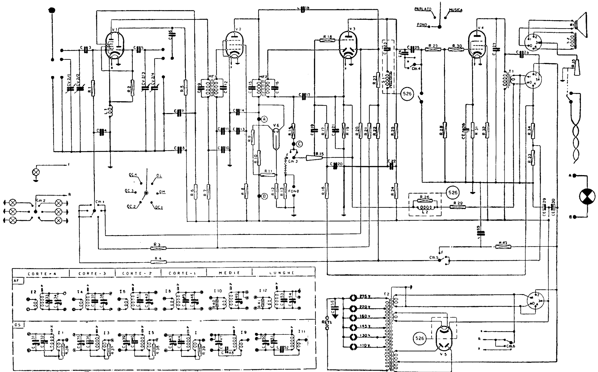
VOCE DEL PADRONE - Mod. 506 e 526 - Variatore di gamma a tamburo rotante con elementi scomponibili. Sei gamme OL, OM e quattro OC. Il mod. 526 è provvisto di WE 12. (Vedere tensioni e taratura a parte).
